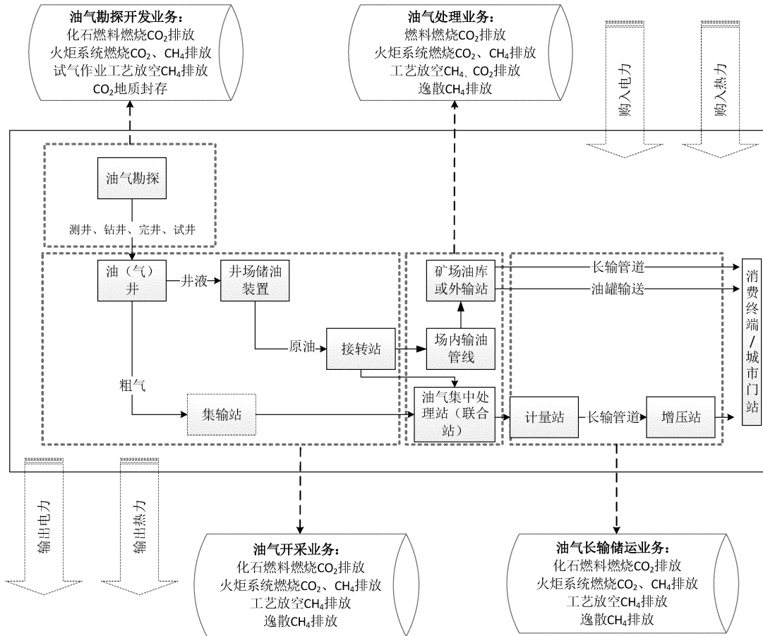
图 A.1 石油天然气生产企业碳排放核算边界示意图
