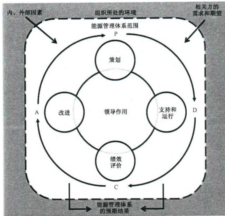
图 1 PDCA 循环
